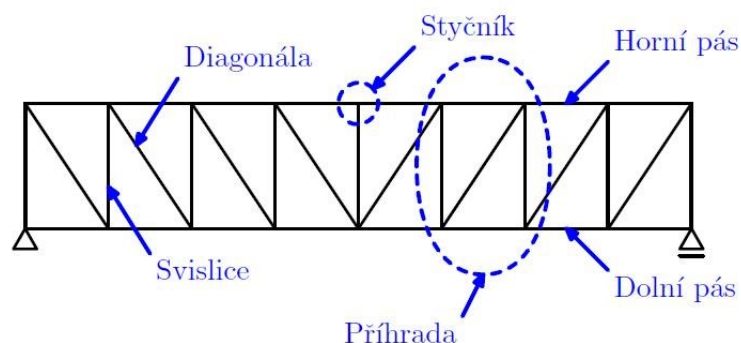
Obr. 28: Příhradová konstrukce
