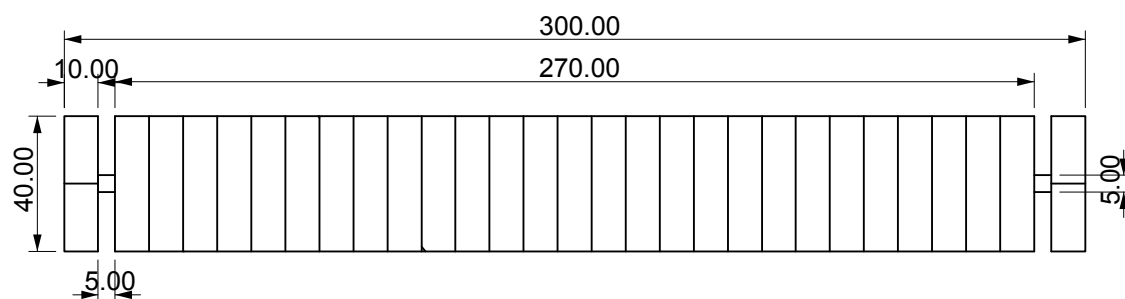
Obr. 36: Půdorys
