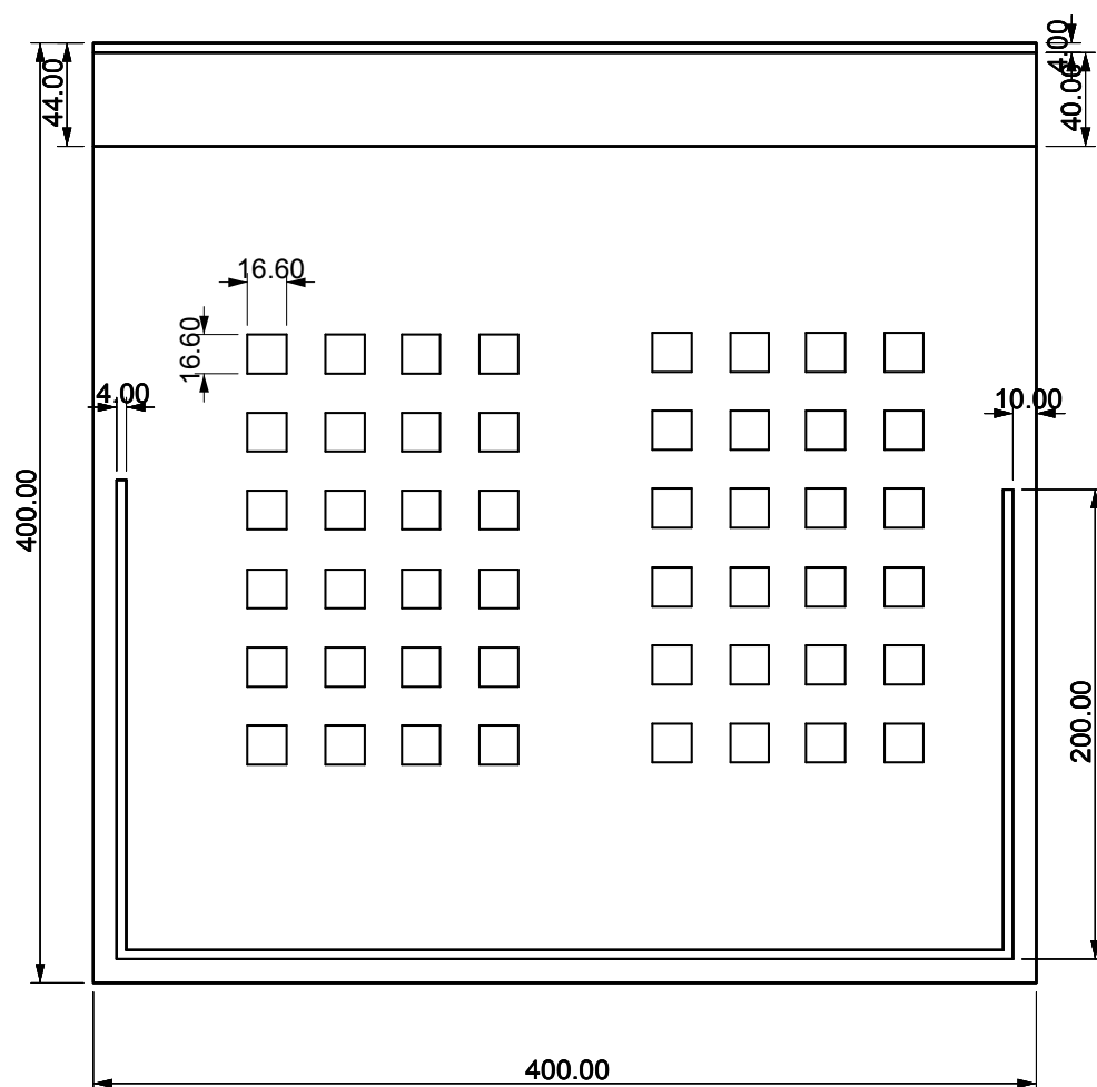
Obr. 38: Půdorys
