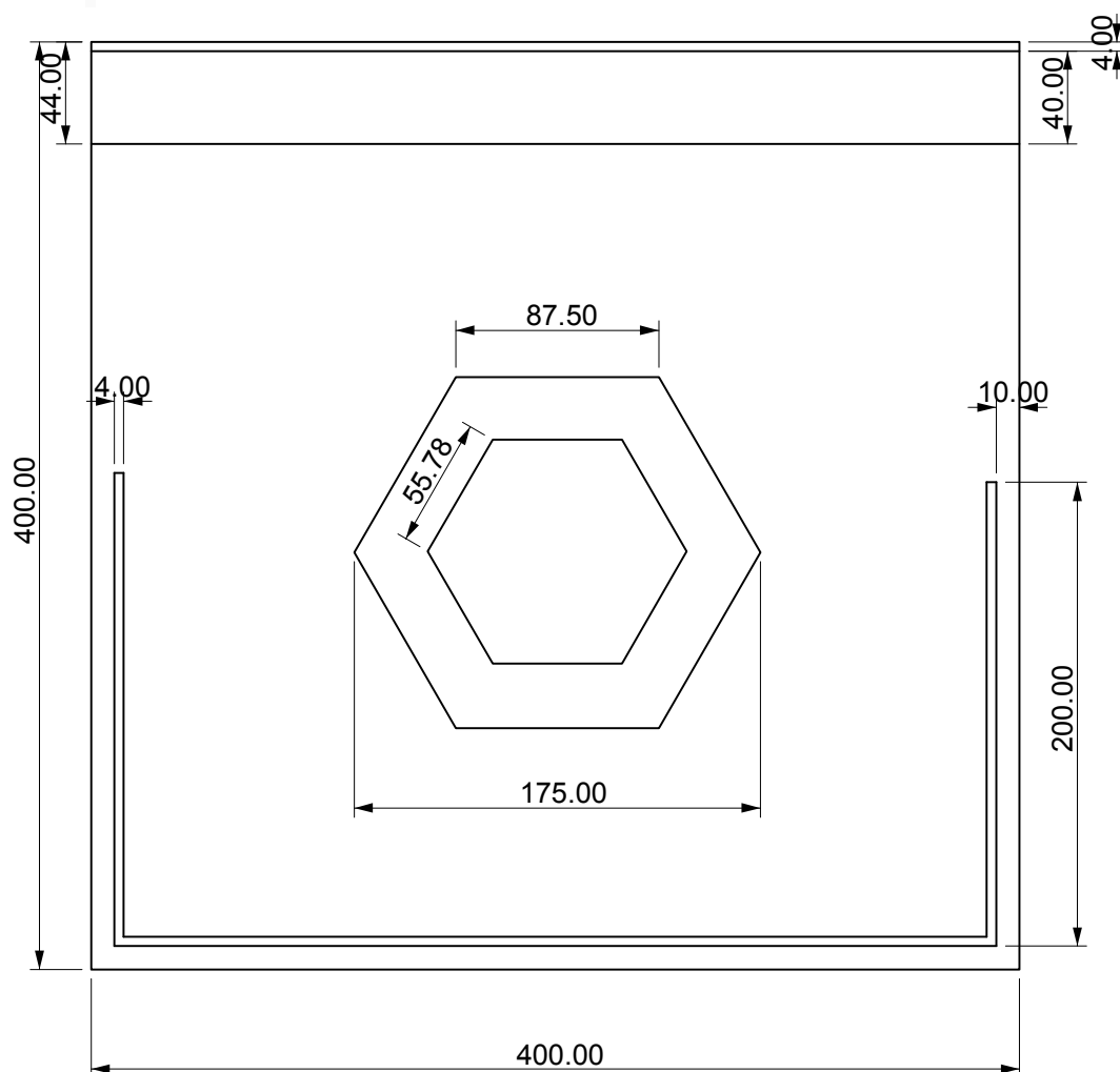
Obr. 35: Půdorys
