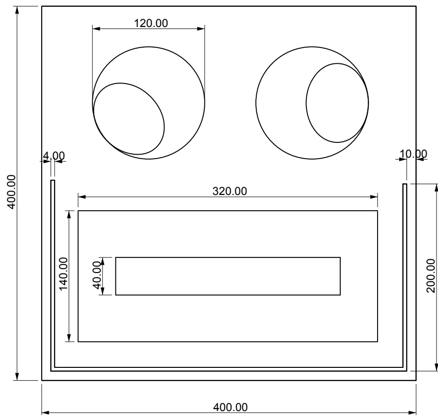
Obr. 41: Půdorys
